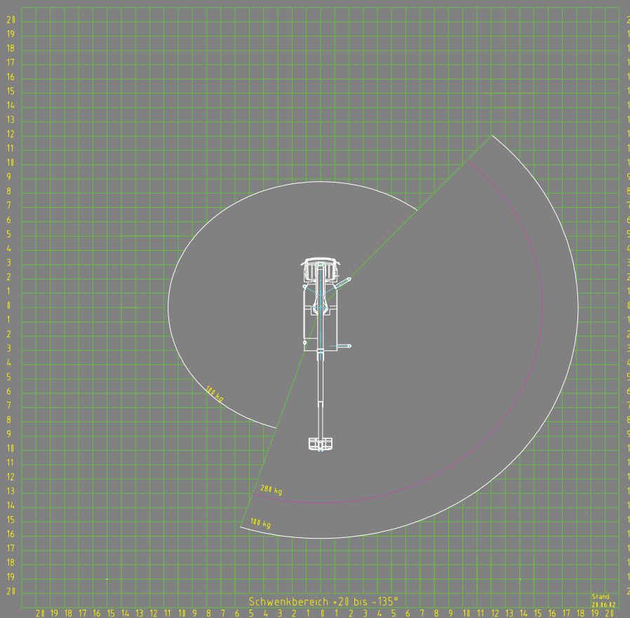
Kennfeld TKA 30 KS einseitige Abstützung
