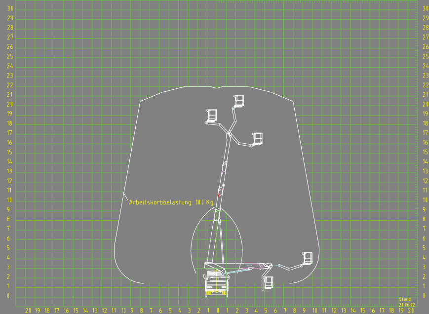
Kennfeld TKA 30 KS schmale Abstützung
