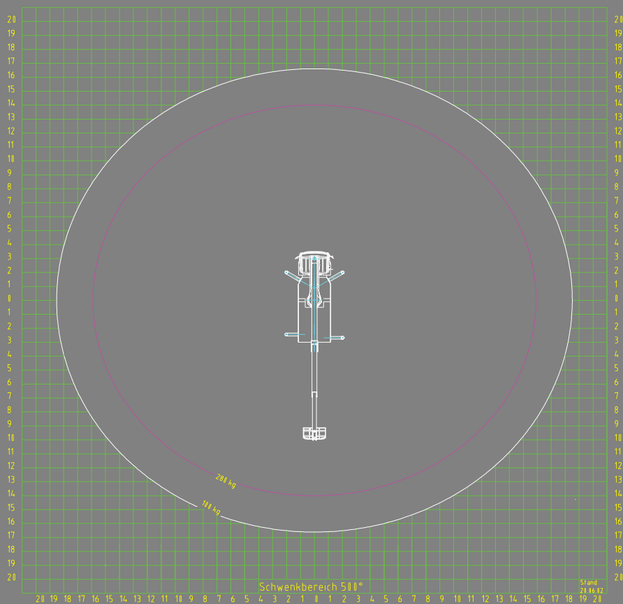
Kennfeld TKA 30 KS breite Abstützung
