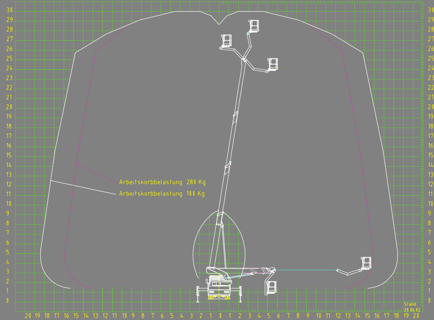
Kennfeld TKA 30 KS breite Abstützung
