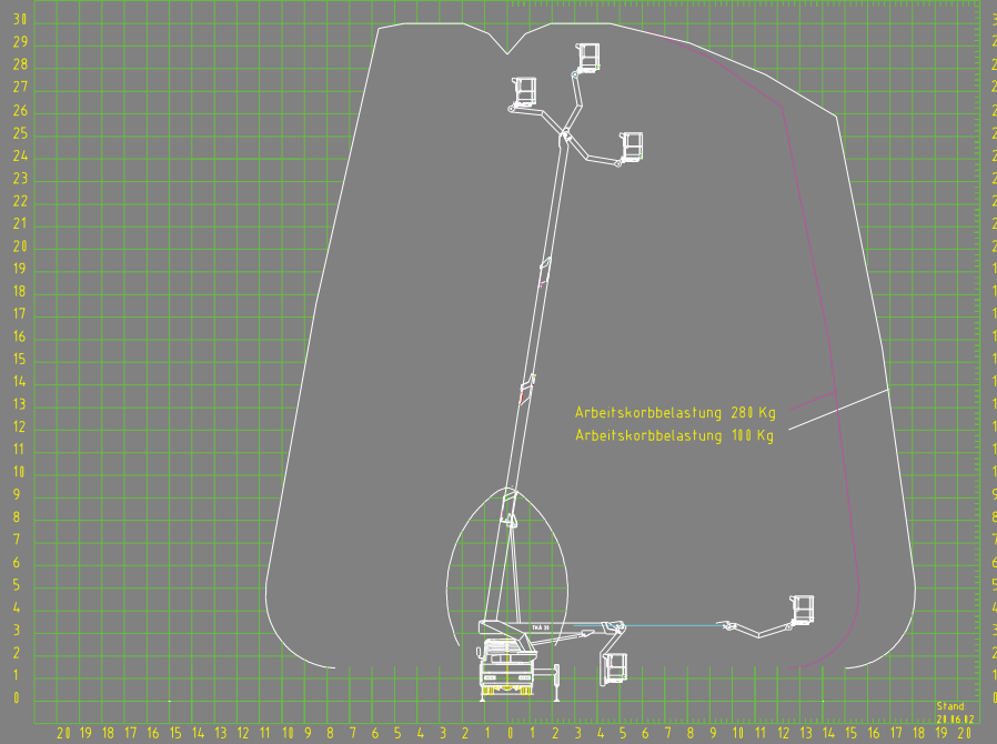
Kennfeld TKA 30 KS einseitige Abstützung
