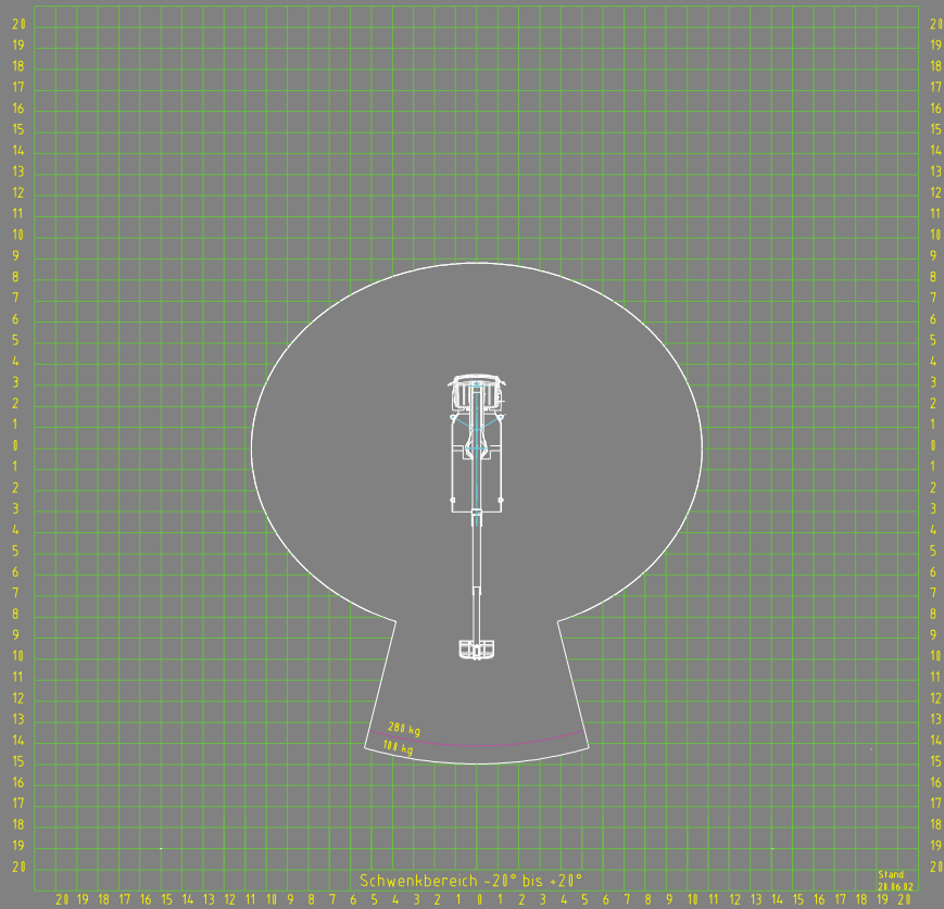
Kennfeld TKA 30 KS schmale Abstützung Höhenbegrenzung 22 m
