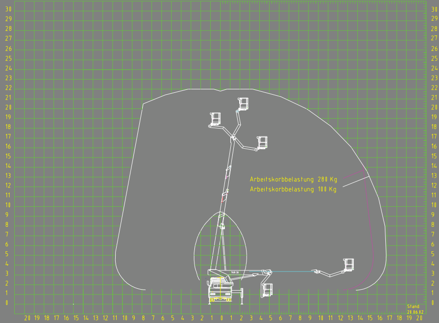
Kennfeld TKA 30 KS einseitige Abstützung
